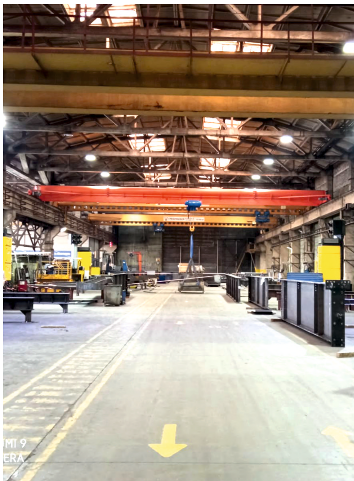
Кран мостовой опорный однобалочный грузоподъемностью 10,0 тонн и длиной пролета 22,5 метров для предприятия в г. Орле.
