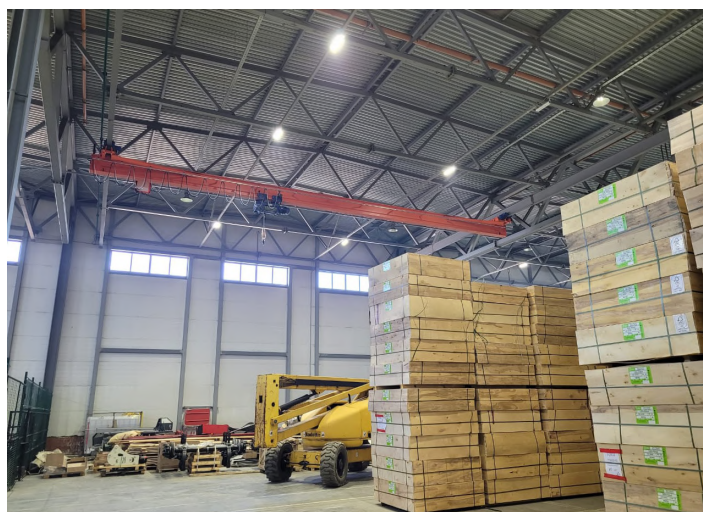
Кран мостовой подвесной грузоподъемностью 5,0 тонн и длиной пролета 18,0 метров для предприятия в г. Санкт-Петербурге.
