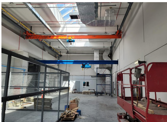
Кран мостовой подвесной однопролетный с электроприводом грузоподъемностью 2,0 тонны, длиной пролета 10,3 метров и монорельс грузоподъемностью 3,2 тонны с полной длиной пролета в 17,0 метров для предприятия в г. Нижнем Новгороде.
